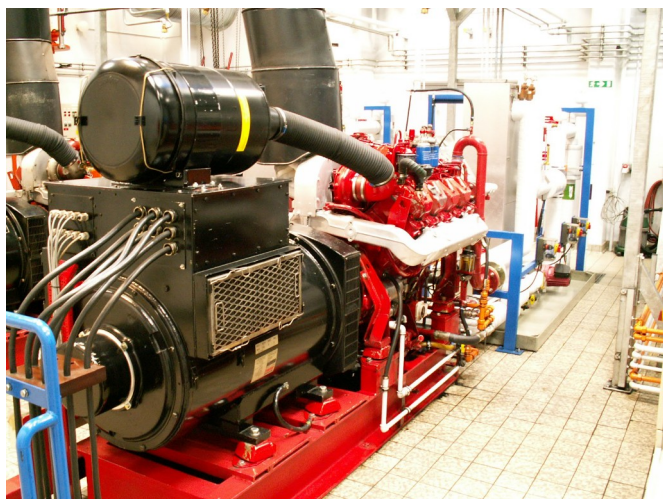
Her er én af de fire store dieselmotorer der forsyner byen.
